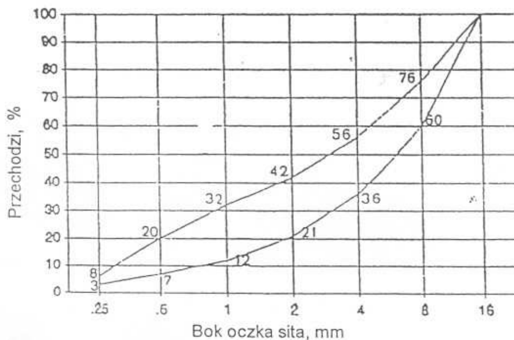
Rysunek 1. Krzywe graniczne uziarnienia kruszywa do betonu
