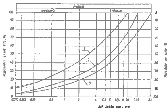
Rysunek 1. Pole dobrego uziarnienia kruszywa przeznaczonych na podbudowy (fundamenty) wykonywane metodą stabilizacji mechanicznej 1-3 kruszywo na podbudowę pomocniczą (fundament)
