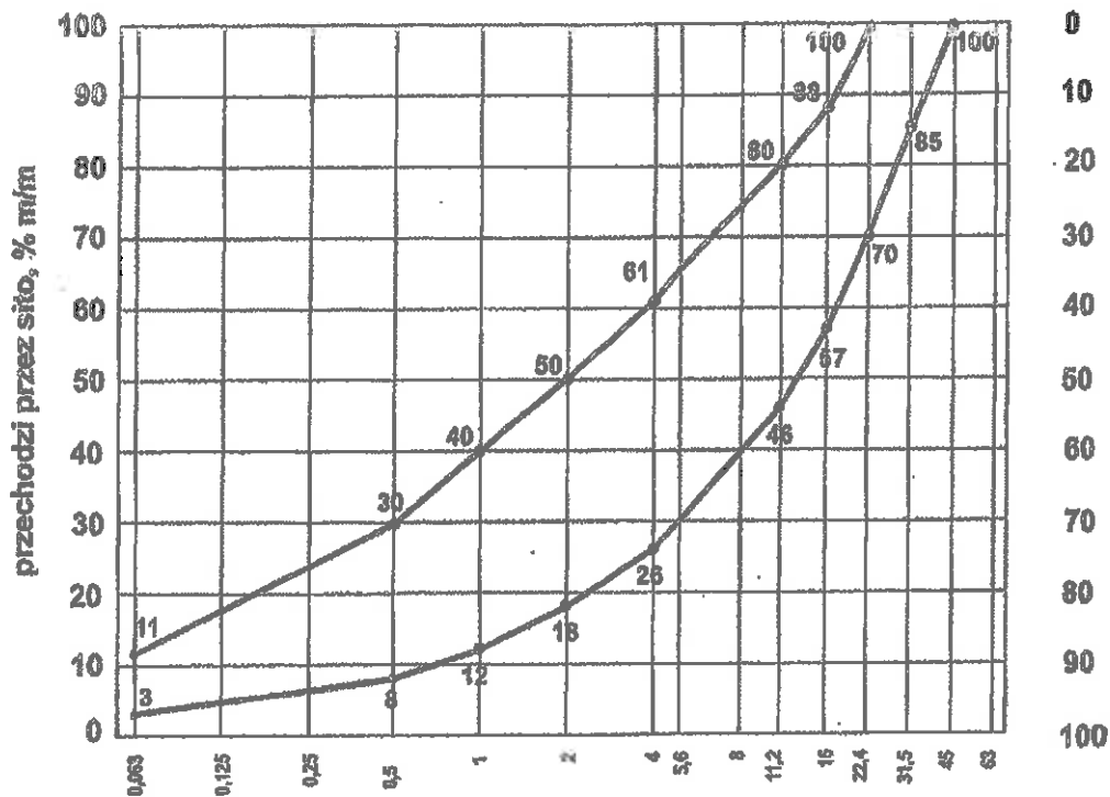
Rys.1 Krzywe uziarnienia mieszanki CBGM 0/31,5
