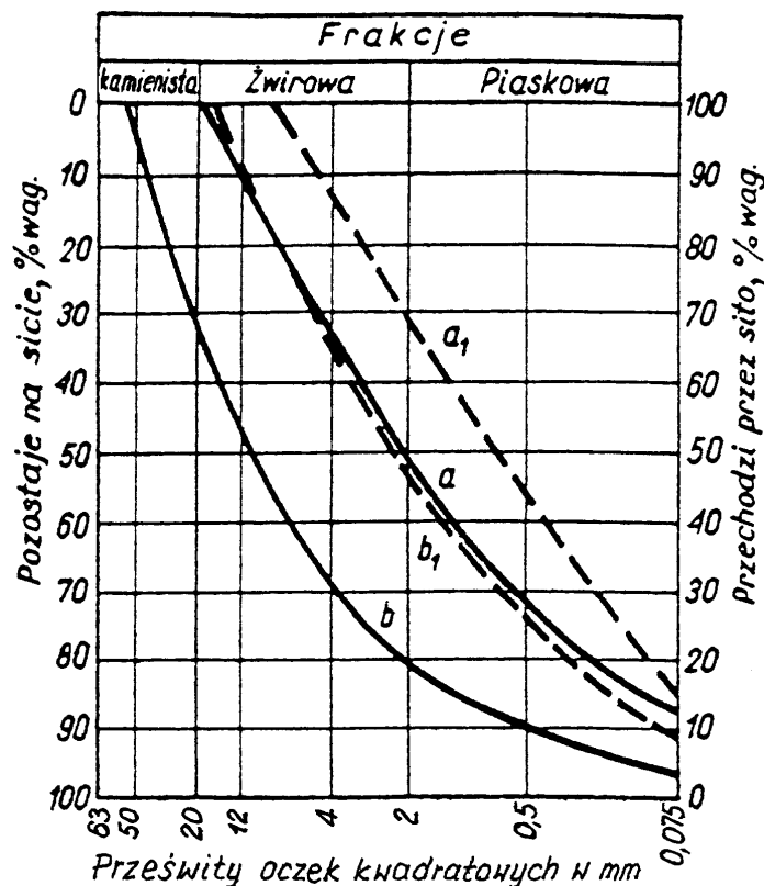
Rysunek 1. Obszar uziarnienia optymalnych mieszank żwirowych
